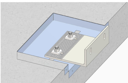
Cajeado JORDAHL® y rail de anclaje después del homigonado
