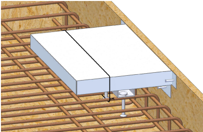
Cajeado JORDAHL® y rail de anclaje antes del hormigonado
